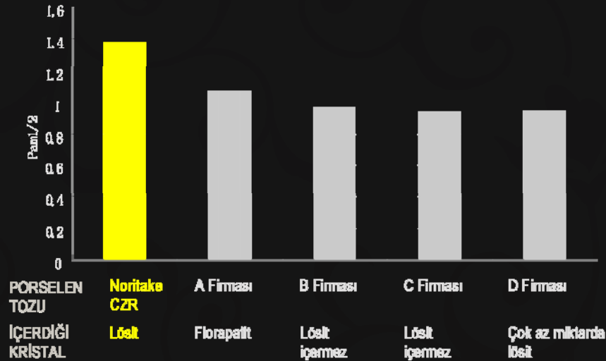
Zirkonya Altyapı Üzerine Uygulanan ZİRKONYA PORSELENİ KIRILMA DİRENCİ (Fracture Toughness) (IF method / JIS R1607) 2008,07,15 NDS Test Result
